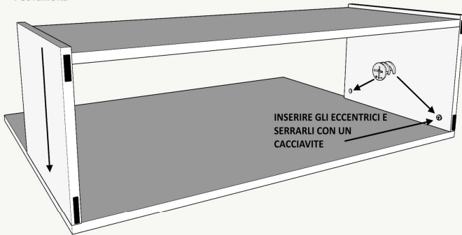
INCASTRARE LA PARTE ASSEMBLATA AL PANNELLO POSTERIORE
